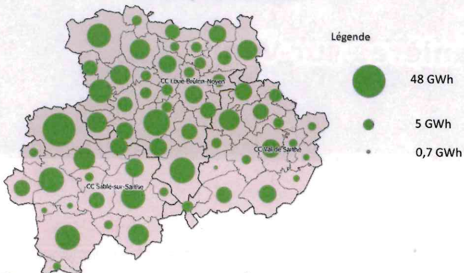
Potentiel de production de chaleur issue du biogaz sur le Pays Vallée de la Sarthe
